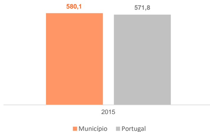
Emissão de CO 2 por município (t/km 2 )
